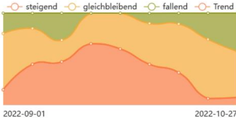
Abbildung 13: Veränderung der SARS-CoV-2-Viruslast im Abwasser, Standorte mit steigendem, gleichbleibendem oder fallendem Trend (Datenstand: 10.10.2022, Quelle: Pandemieradar https://www.rki.de )
