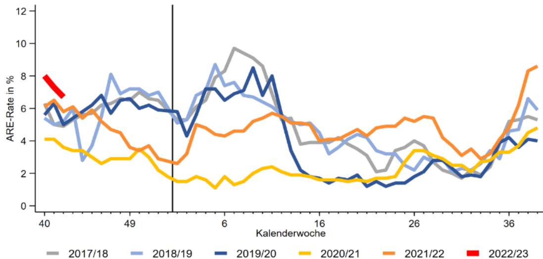
Abbildung 11: Vergleich der für die Bevölkerung in Deutschland geschätzten ARE-Raten (in Prozent) in den Saisons 2017/18 bis 2022/23 (ab der 40.KW 2022). Der senkrechte Strich markiert den Jahreswechsel (Quelle: RKI).
