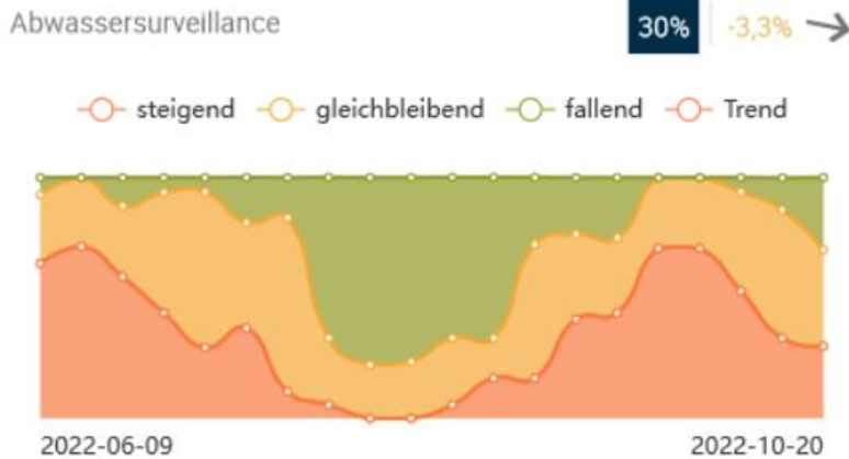
Abbildung 13: Veränderung der SARS-CoV-2-Viruslast im Abwasser, Standorte mit steigendem, gleichbleibendem oder fallendem Trend (Datenstand: 27.10.2022, Quelle: Pandemieradar https://www.rki.de )
