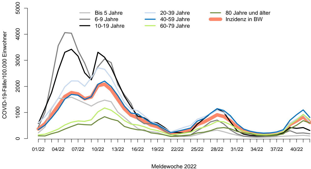
Abbildung 4: Übermittelte COVID-19-Fälle in 2022 pro 100.000 Einwohner, Baden-Württemberg, nach Altersgruppe und Meldewoche mit Landesdurchschnitt (rote Linie), Stand: 27.10.2022, 16:00 Uhr.
