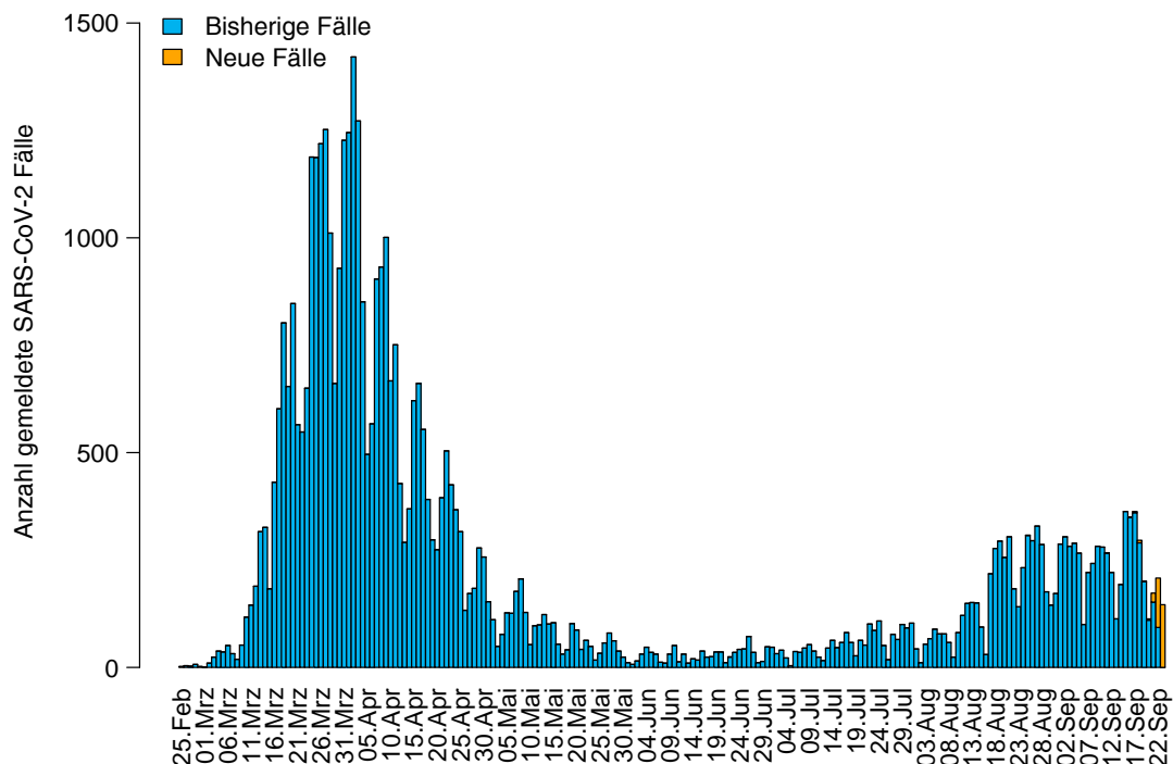
Abb.1: Anzahl der an das LGA übermittelten SARS-CoV-2 Fälle nach Meldedatum (blau: bisherige Fälle; gelb: neu übermittelte Fälle), Baden-Württemberg, Stand: 23.09.2020, 16:00 Uhr.
