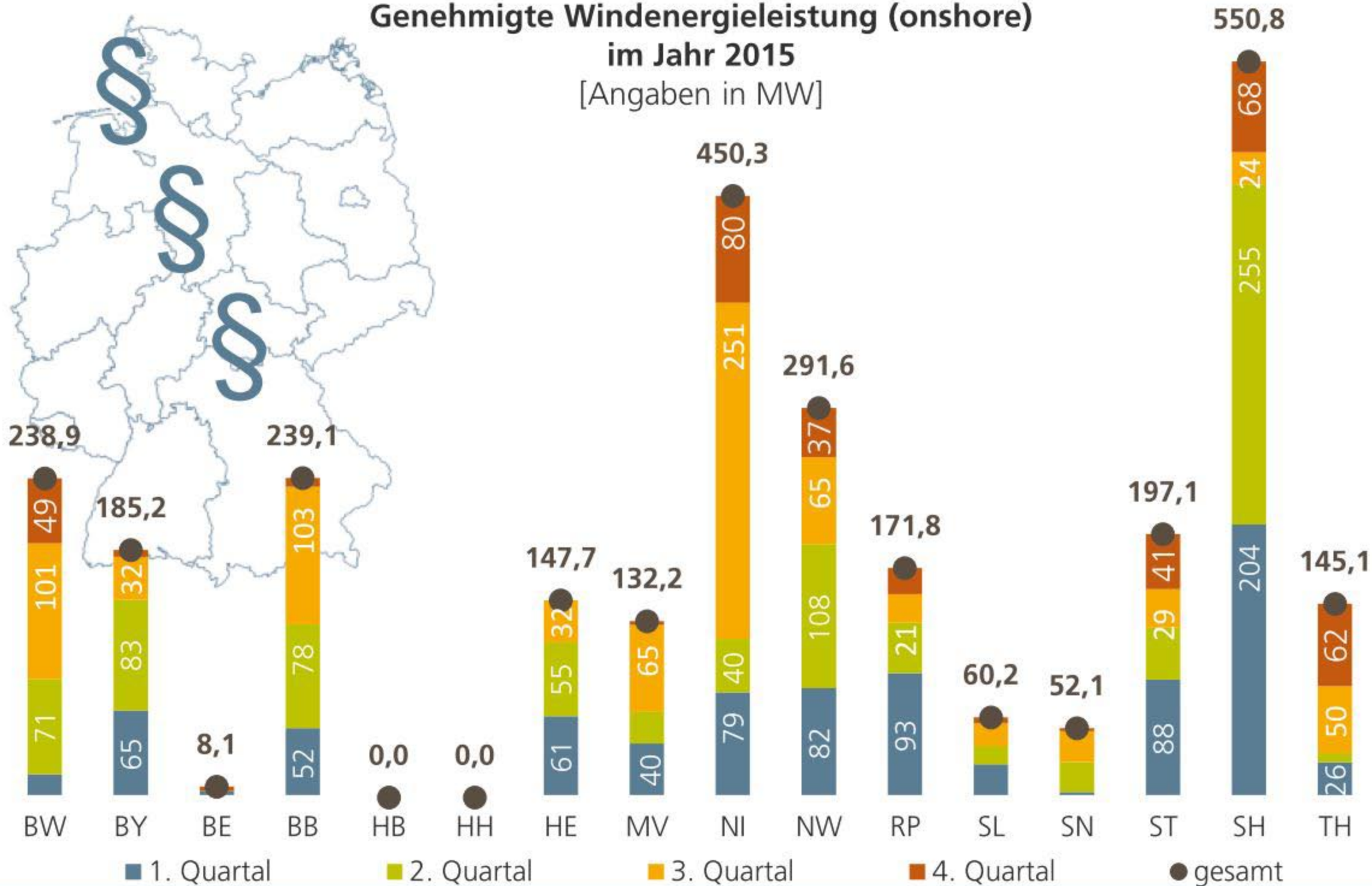
Abbildung 4: In den Bundesländern neu genehmigte Windenergieleistung; Daten: BNetzA, Auswertung und Graphik: FA Wind
